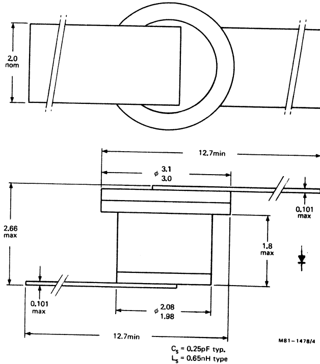
case style MO-66
