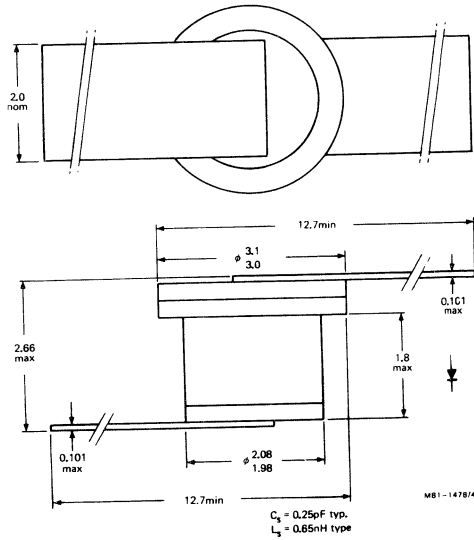
case style MO-66
